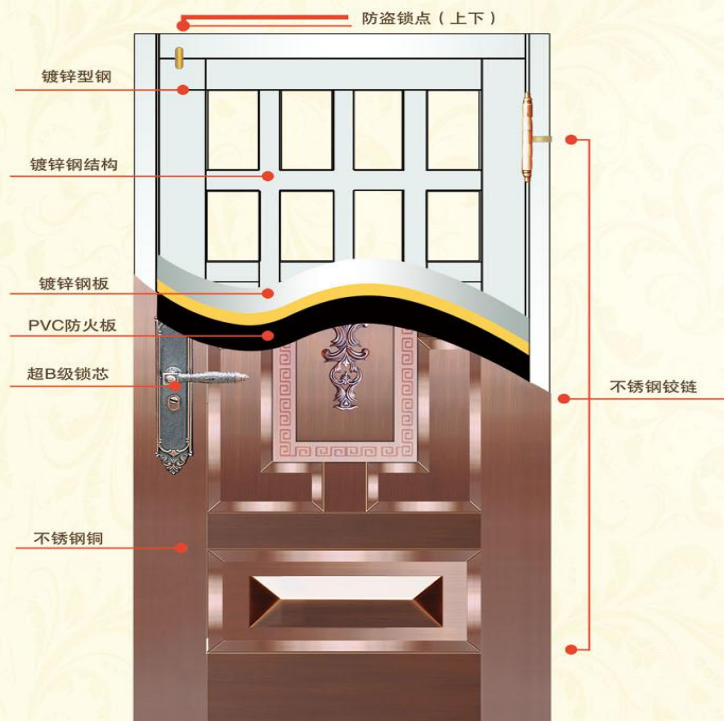
结构示意图
